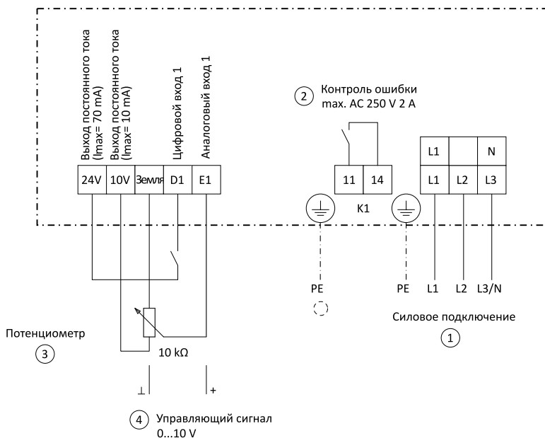
Схемы подключений электродвигателей вентиляторов (рис. 7)
