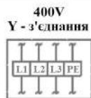
Клемна коробка
