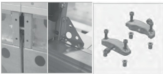
З'єднання рам та секцій (рис. 6)
