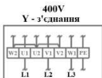
Клемна коробка
