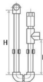
Расчёт высоты сифона (рис. 12)
