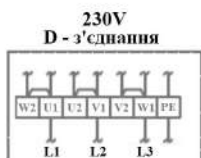
Клемна коробка
