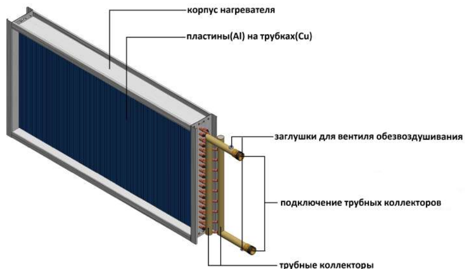
Конструкция нагревателя (рис. 8)
